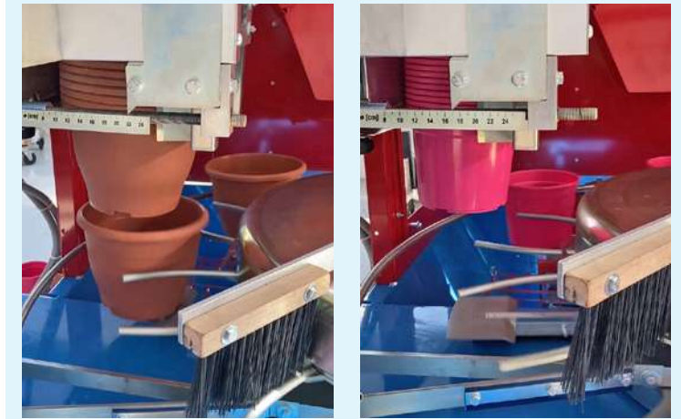
Llenadora IA3500 con cabezal individual : es capaz de trabajar con macetas de 8 a 27 cm , de diferentes formas y materiales.
