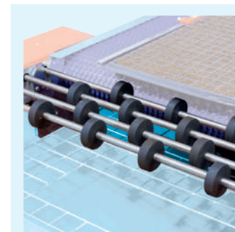
58 Transportador de salida motorizado, con 4 filas de rodillos.
