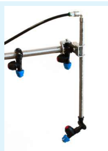
Ugello indipendente snodato con prolungamento in acciaio inox regolabile in altezza, completo di valvola per irrigazione bordi .
