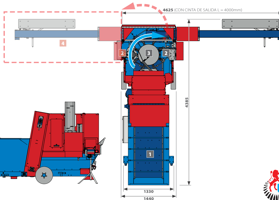
Cinta de alimentación de macetas, combinado a un cabezal doble para macetas cuadradas (accesorio).
